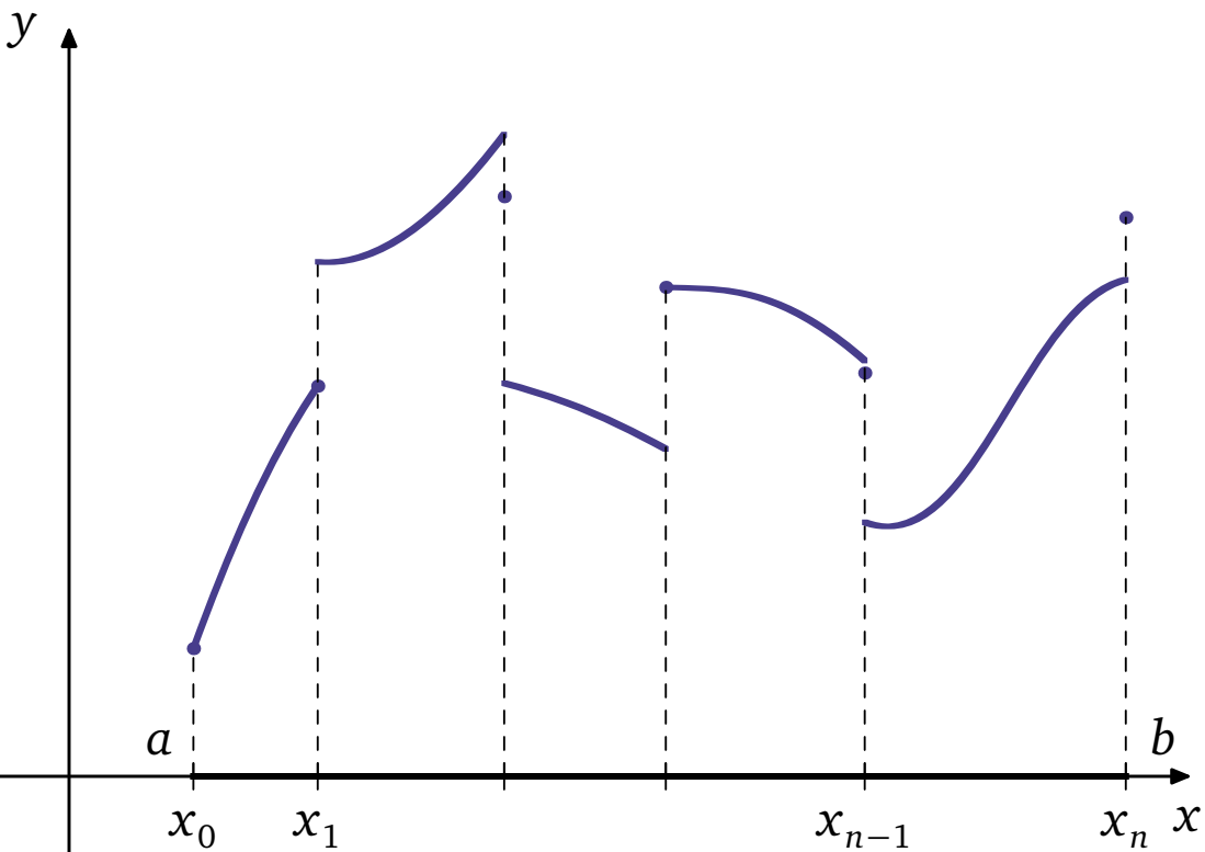
Fonction continue par morceaux sur un segment.
