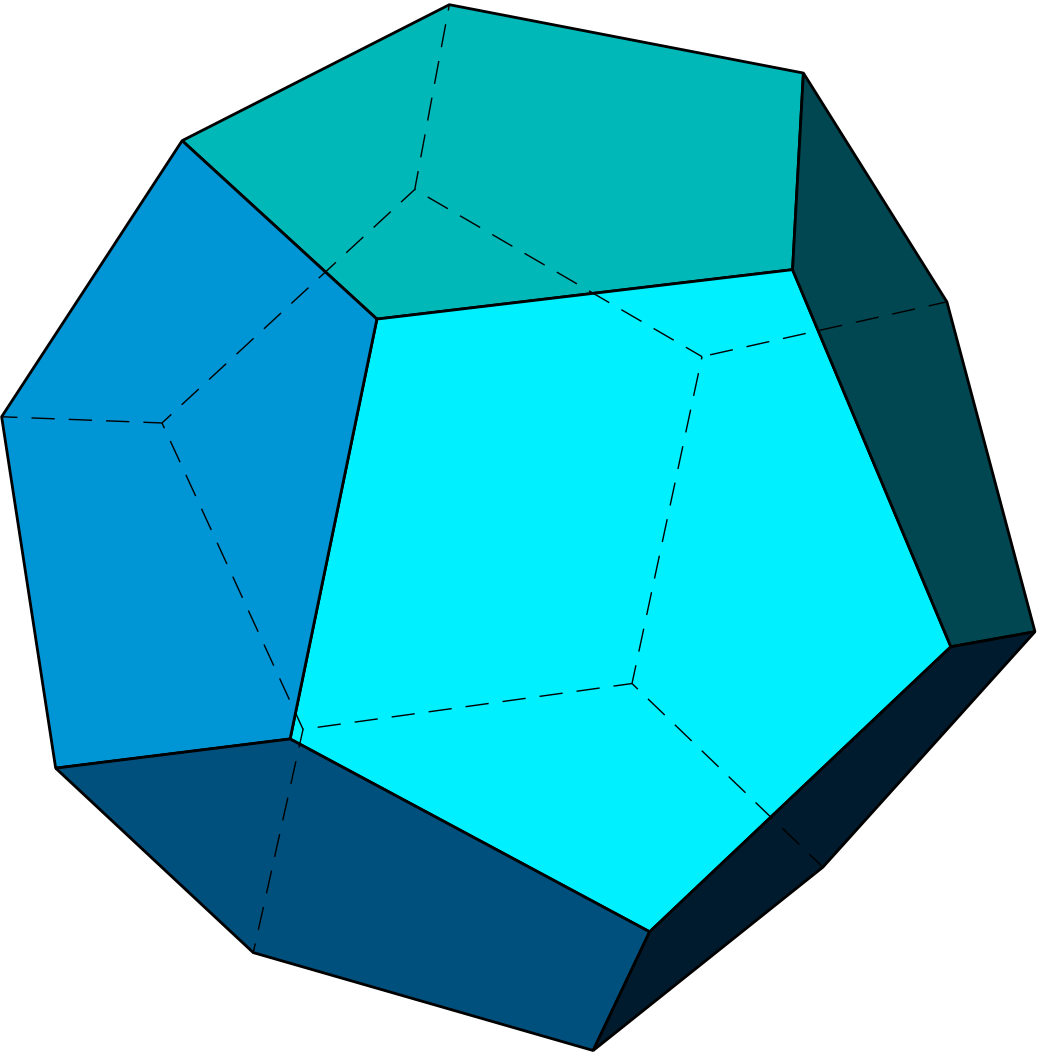
Dodécaèdre
