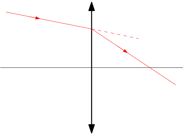
Lentille convergente
