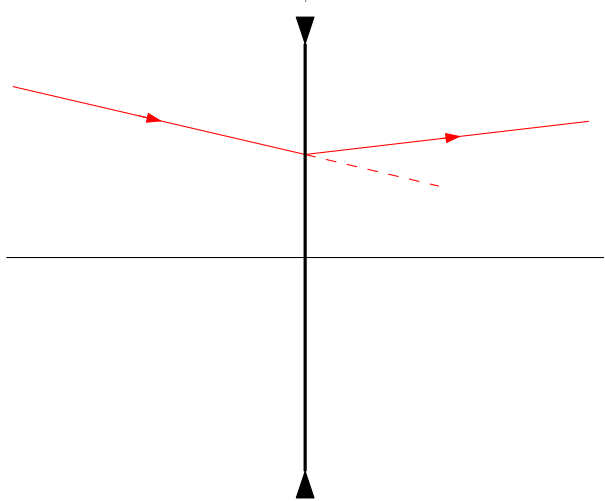
Lentille divergente
